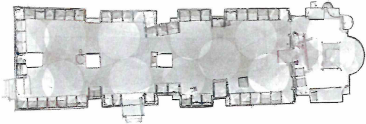
Κάτοψη του Ναού όπως αυτή αποτυπώθηκε με τη χρήση 3D Scanner
